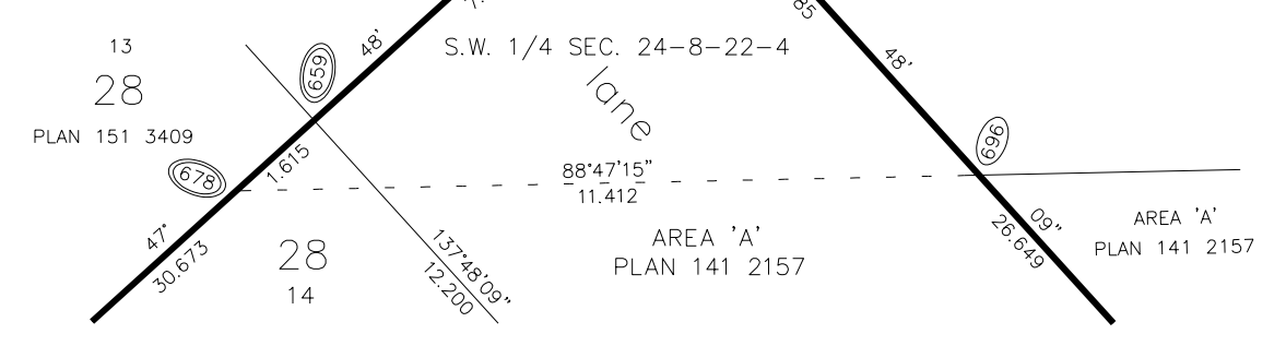
DETAIL 'B' 1:100
